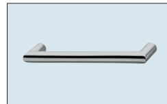
Nr. 705 Metallbügelgriff Edelstahl-Optik Bohrabstand 160 mm Überstand nach vorn: 41 mm
